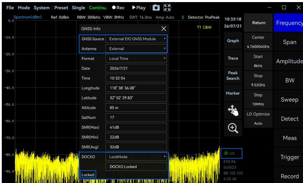
figure 6 Use the External EIO GNSS Module
