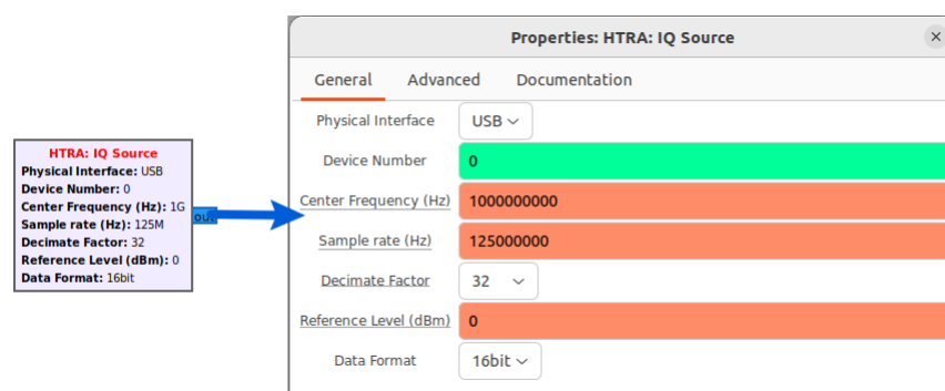
Figure 10 HTRA: IQ Source Module Parameter Description
